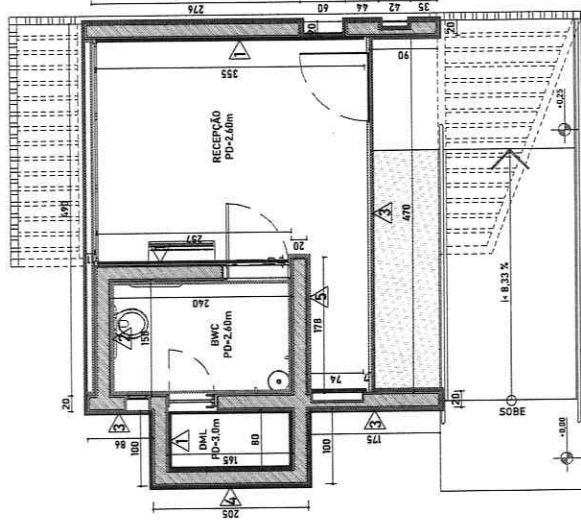
PLANTA BAIXA - REVESTIMENTO PAREDES Esc. 1/50
