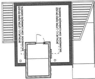
PLANTA BAIXA RESERVATÓRIO Esc. 1/75
