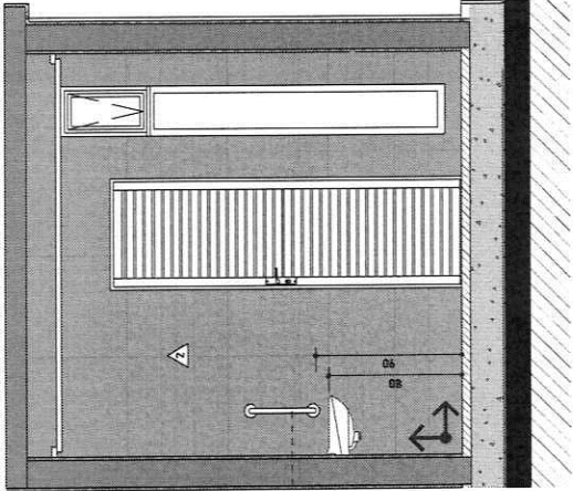
VISTA 04 BANHEIRO PcD - PAGINAÇÃO
