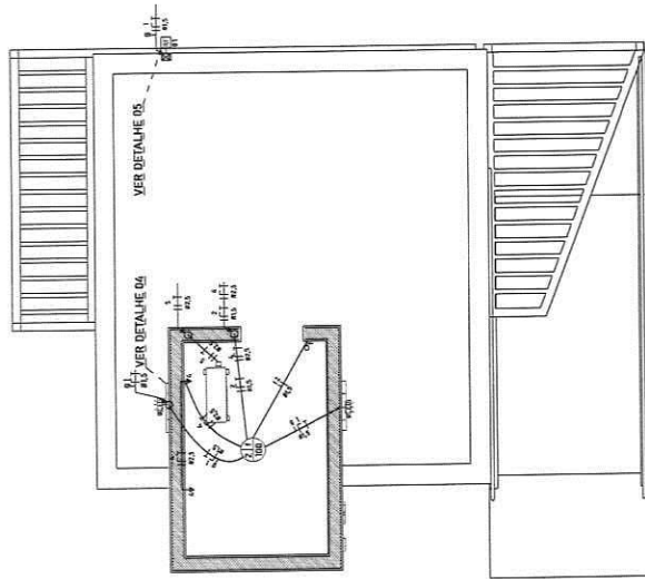
PLANTA BAIXA - RESERVATÓRIO Esc. 1:50
