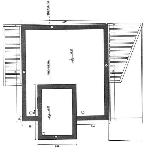
PLANTA DE COBERTURA - PINGADEIRAS Esc. 1/50
