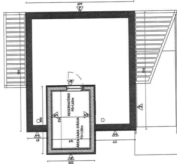
PLANTA BAIXA RESERVATÓRIO - REVESTIMENTO PAREDES Esc. 1/50
