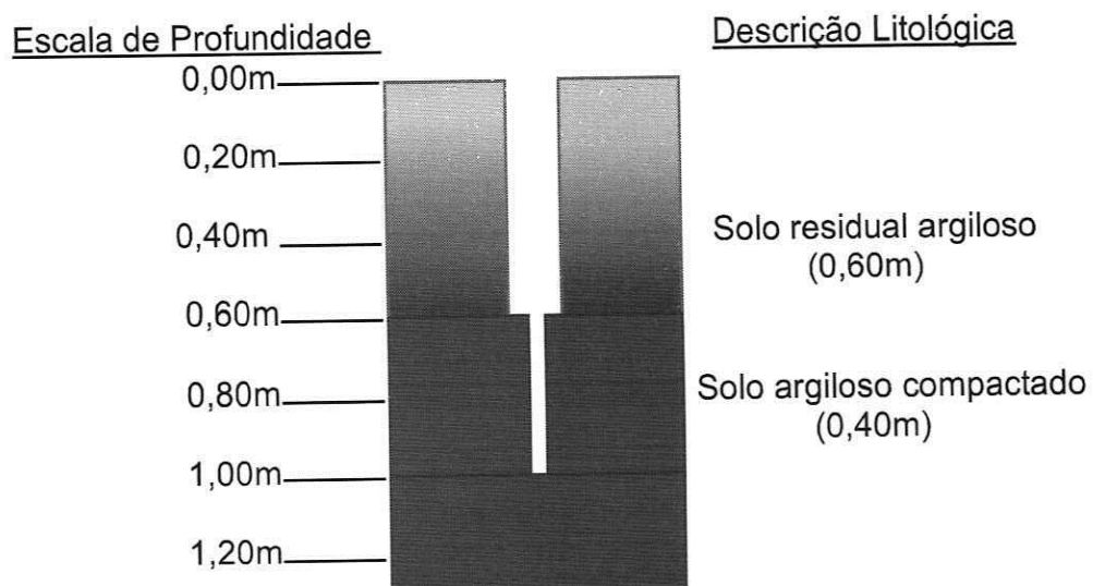
Fig. 13: Perfil Geológico esquemático em ST 13 com Profundidade Final 1,50m.
