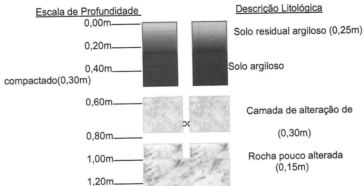
Fig. 11: Perfil Geológico esquemático em ST 11 com Profundidade Final 1,00m.
