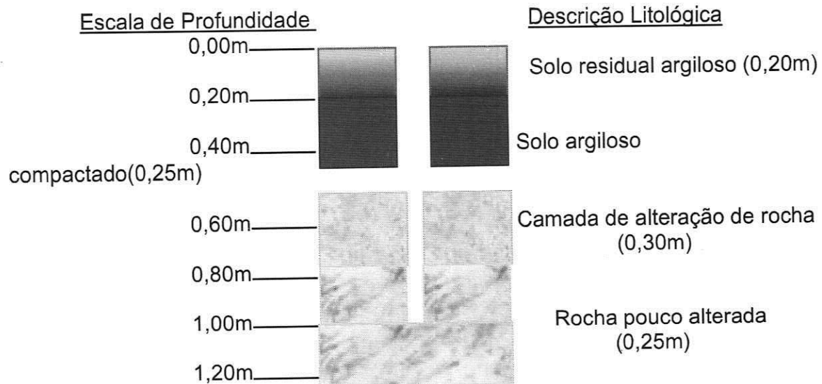
Fig. 16: Perfil Geológico esquemático em ST 16 com Profundidade Final 1,00m.
